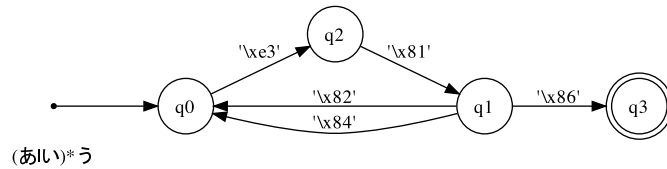
図 6 正規表現 “(a|i)*u” に対応する DFA
