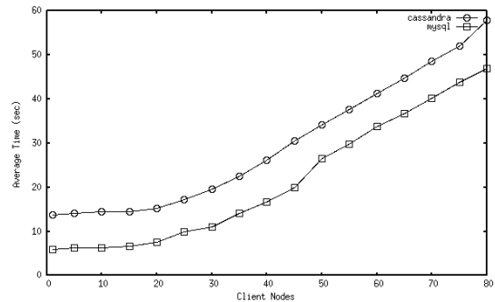
図 3 サーバー 1 上でのベンチマーク (Read)
