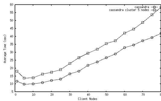
図 8 サーバー 1 を複数ノードにしたベンチマーク (Write)
