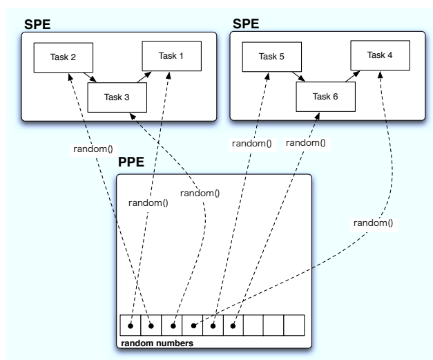
図 6 PPE 内での乱数の生成と乱数の受け渡し
