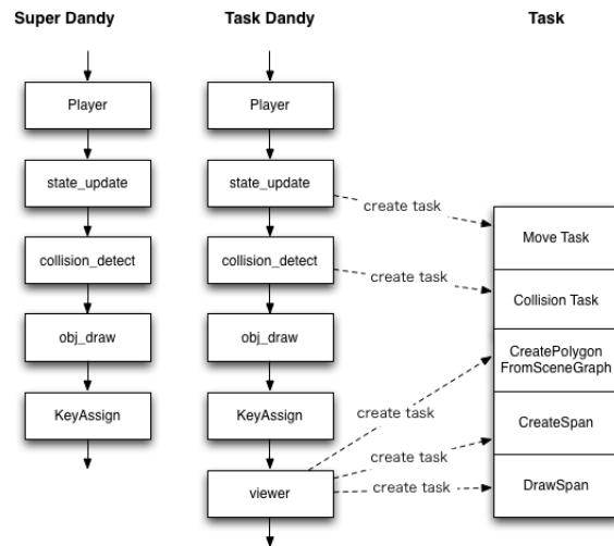
図 4 Super Dandy と Task Dandy の処理
