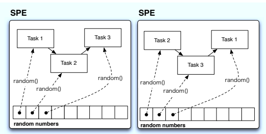
図 2 SPE 内での乱数の生成
