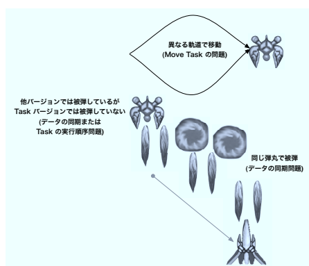
図 5 Task Dandy で起こりうるバグ
