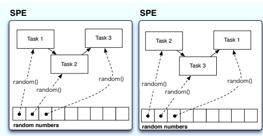
図 2 SPE 内での乱数の生成
