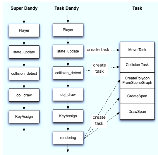
図 4 Super Dandy と Task Dandy の処理
