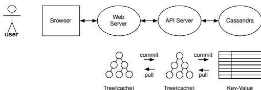
図 9 多段キャッシュとマージ処理
