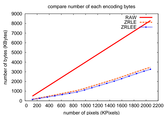
図 6 RAW,ZRLE,ZRLEE による 1 画面 (1920*1080) 描画にかかるデータ量。x 軸はピクセル数、y 軸はバイト数を表している。
