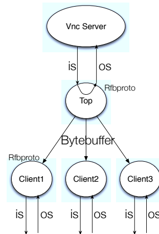
図 3 クライアントへは並列にデータを送信する。
