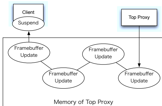
図 4 クライアントサスペンド時の Top のメモリの様子。 データが残る続けメモリを圧迫してしまう。
