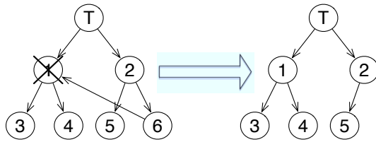
図 2 番号の一番大きいノードが報告を受け指定された場所 (1 番) に接続を行う。(T は Top)
