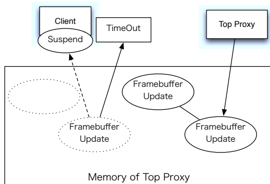
図 5 TimeOut が代わりにデータを取得する
