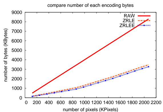
図 5 RAW, ZRLE, ZRLEE による 1 画面描画にかかるデータ量
