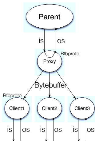
図 2 Vnc server(Parent) から受け取ったデータを自身に繋がっているクライアントへ送信する。クライアントは次のクライアントへデータを送信する。
