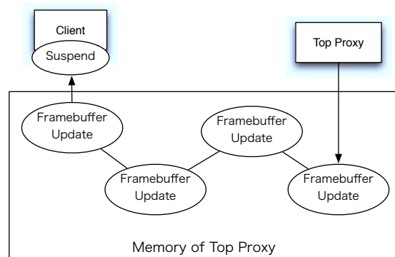
図 3 クライアントサスペンド時のトップのメモリ
