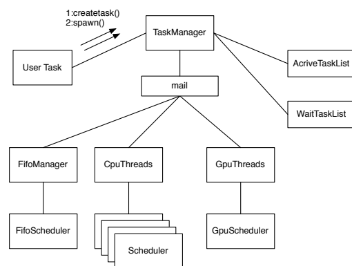
図 1 Task Manager
