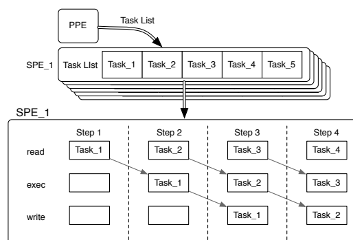
図 3.2: Task Scheduler
