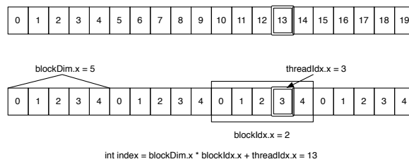
図 2.5: Calculate Index
