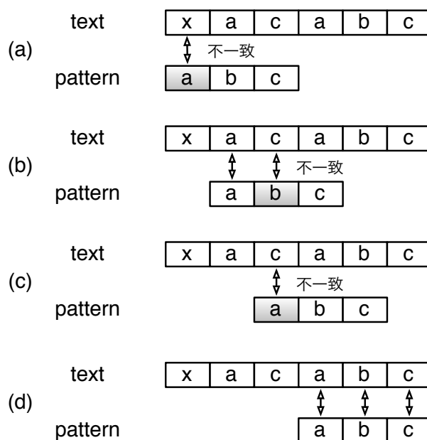
図 3.1: 力まかせ法
