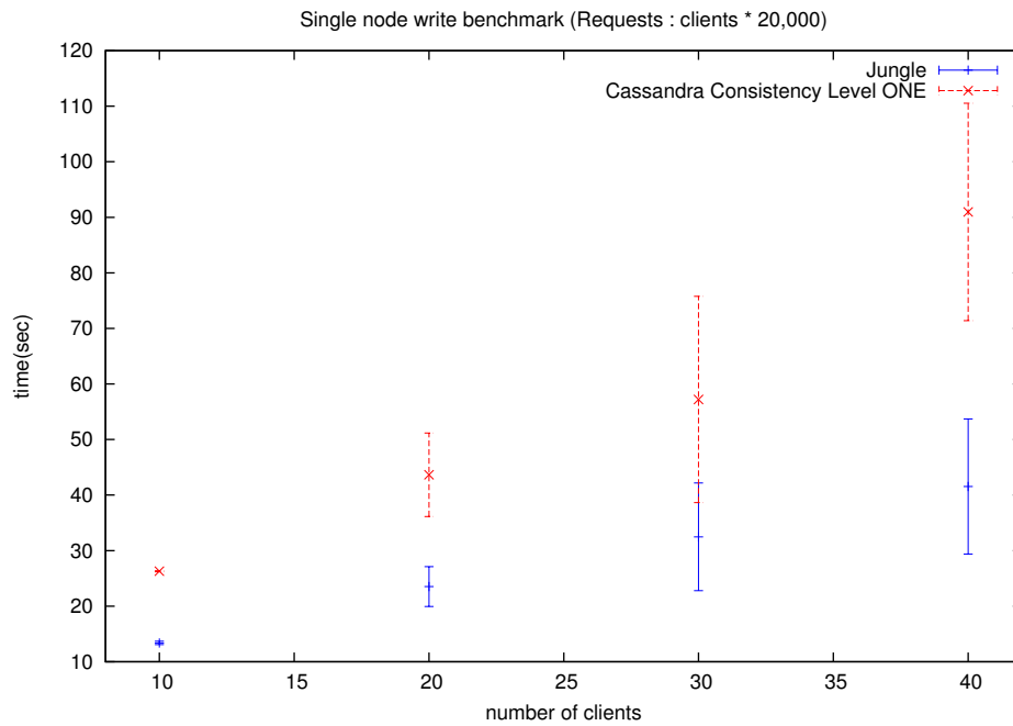
図 6.5: 複数のクライアントから一台への負荷
