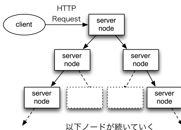
図 6.1: 複数起動中の Jungle の 1 ノードへの負荷
