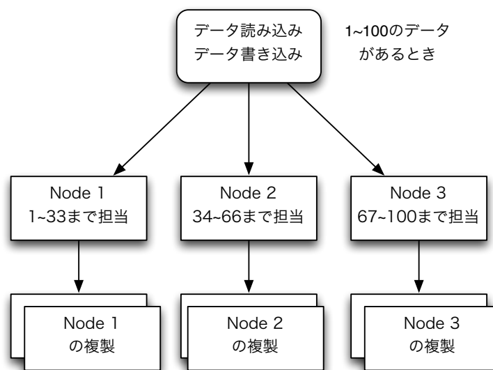
図 2.1: Sharding
