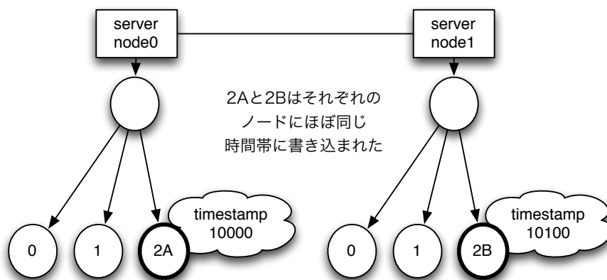
図 4.3: 他サーバノードの編集データ反映による整合性の崩れ 1
