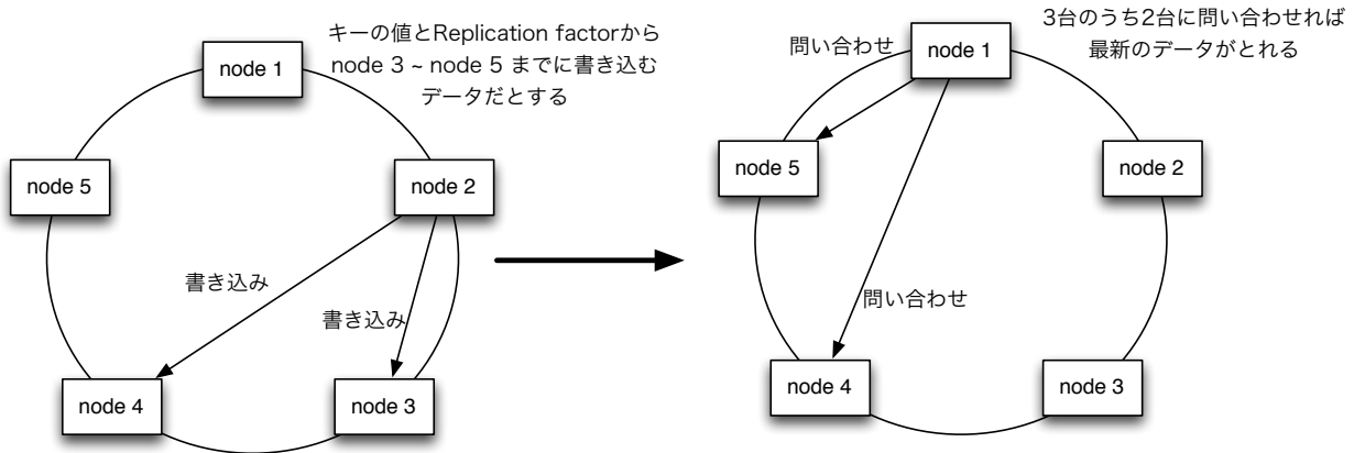
図 2.5: ConsistencyLevel QUORUM による書き込み
