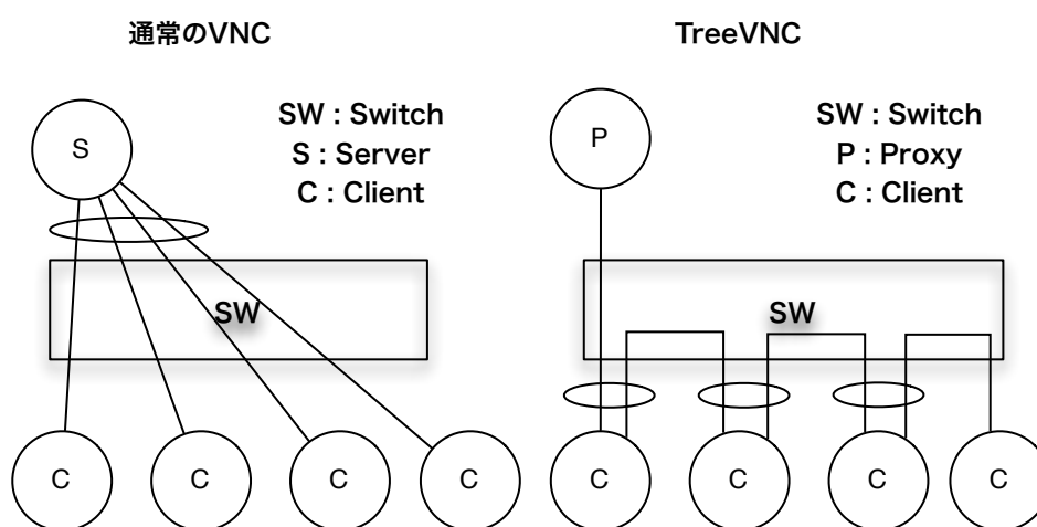
図 3.3: TreeVNC の構造
