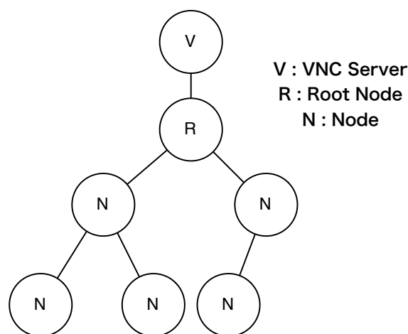
図 3.2: TreeVNC の構造
