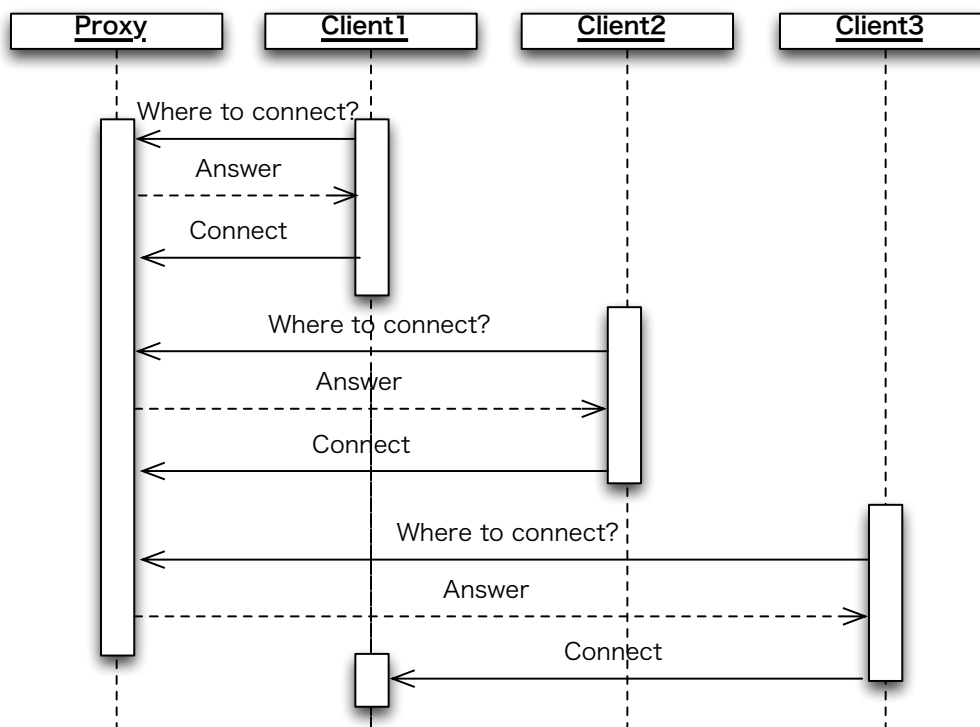
図 3.4: TreeVNC の構造
