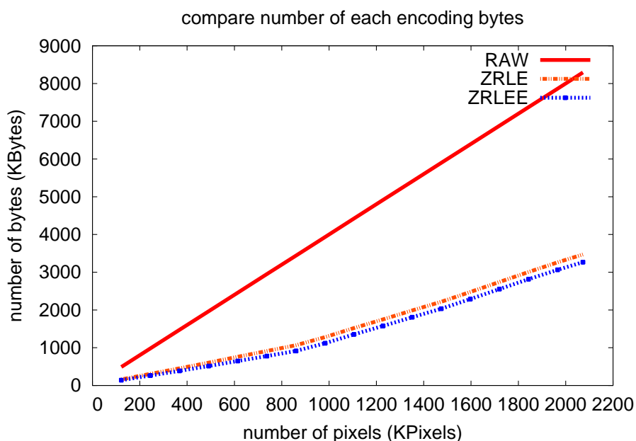
図 6.2: RAW,ZRLE,ZRLEE による 1 画面 (1920*1080) 描画にかかるデータ量。x 軸はピクセル数、y 軸はバイト数を表している。
