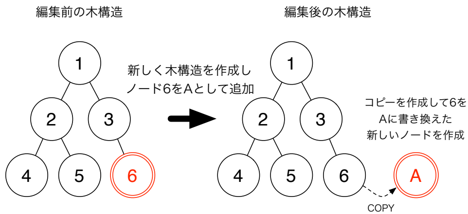
図 3.5: ステップ 2: 変更したいノードをコピーし、コピーしたノードの内容を変更した新しいノードを作成する
