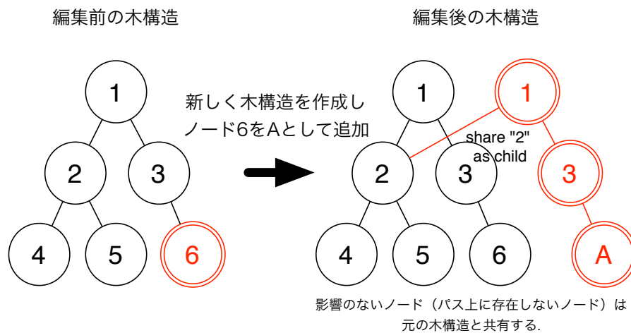
図 3.7: ステップ 4: 影響のないノードは共有する
