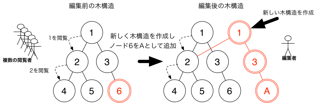
図 3.8: 並列に読み書きが可能な非破壊的木構造
