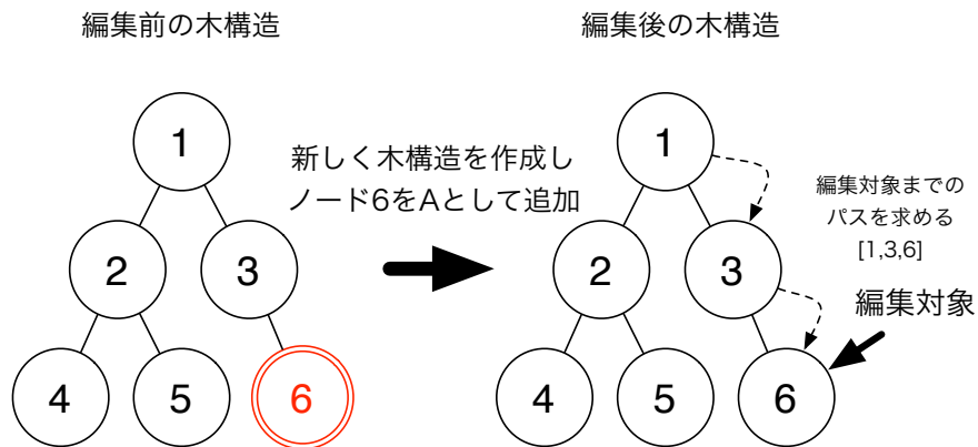
図 3.4: ステップ 1: 変更したいノードまでのパスを求める
