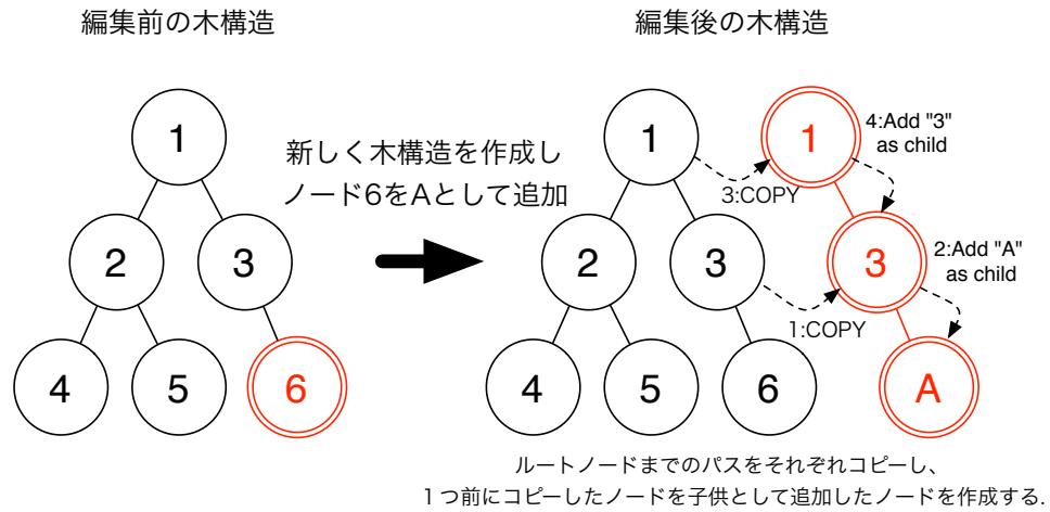
図 3.6: ステップ 3: 求めたパス上に存在するノードをルートノードまでコピーする
