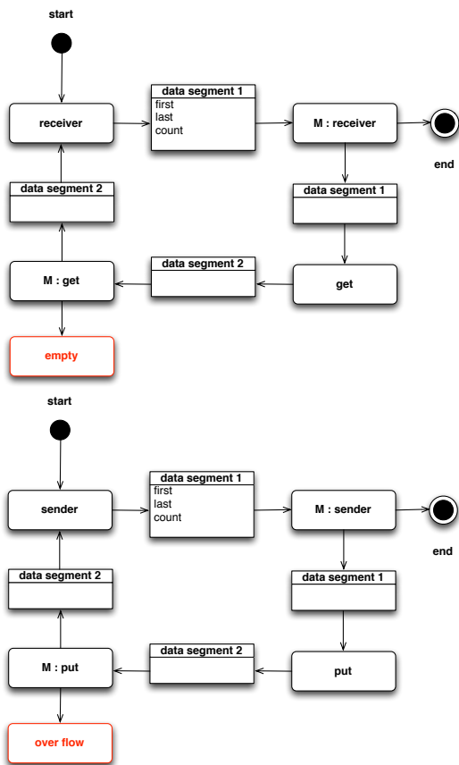
図 3: Synchronized Queue
