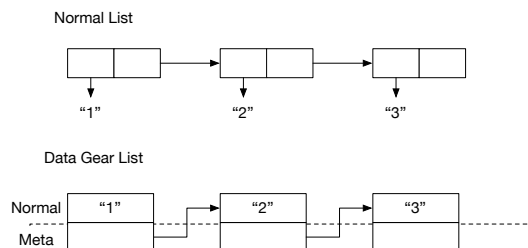
図 2: List の表現
