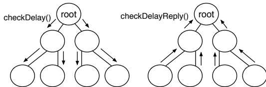
図 6 CHECK_DELAY, CHECK_DELAY_REPLY
