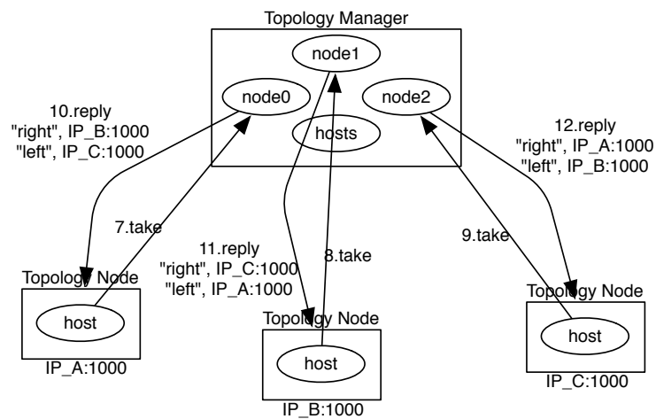
図 3: 参加表明したノードに対して抽象名を返す
