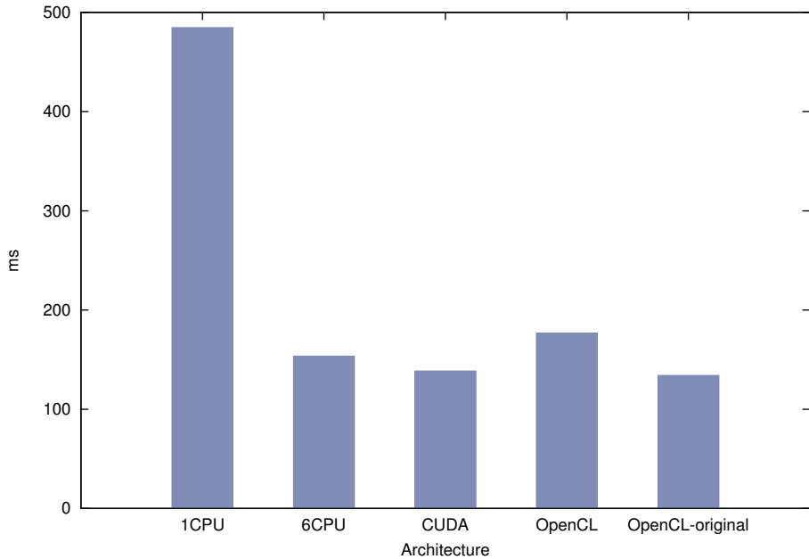
FFT Benchmark
