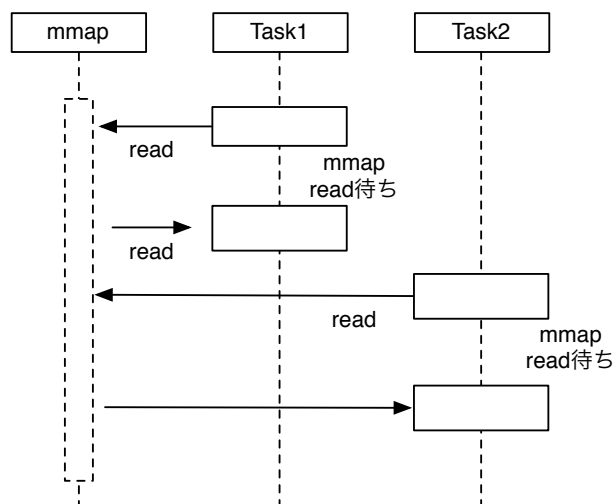
図 7.1: mmap の Model
