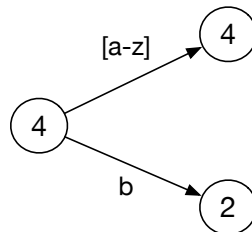
図 4.18: b が入力されるとどちらに遷移すればいいのかわからない
