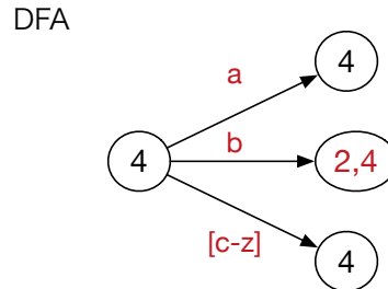
図 4.19: b が入力されたときは新しい状態を作り、新しい状態に遷移させる
