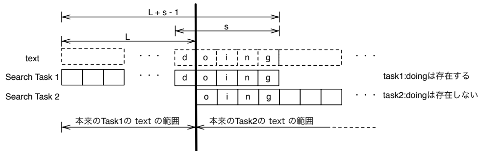
図 4.8: 分割周りの処理
