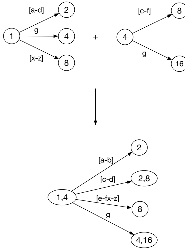
図 4.21: Subset Construction による新しい状態の生成
