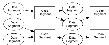
図 1 CodeSegment の依存関係
