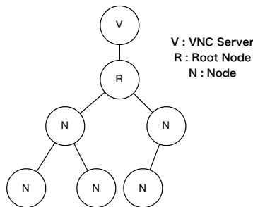
図4 TreeVNC の構造
