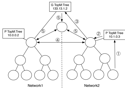
図 8 NAT を越えた接続
