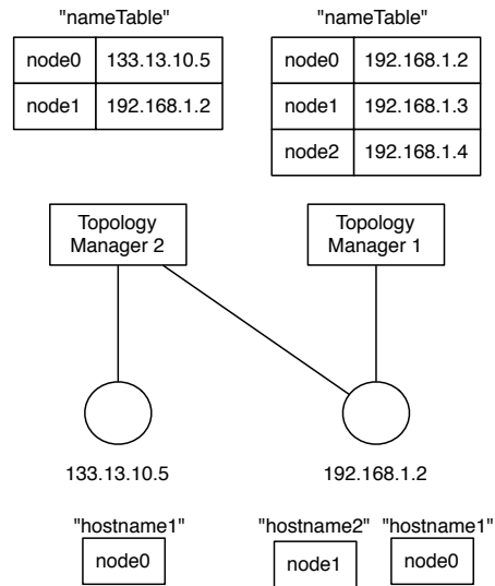
図 7 Topology Node は複数の nodeName を持つ
