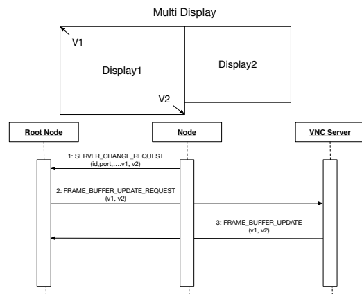
図 2: マルチディスプレイへの対応
