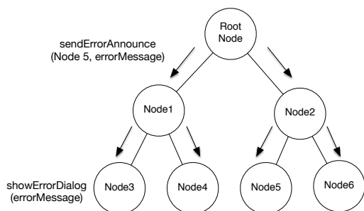
図 3: ERROR_ANNOUNCE メッセージの挙動
