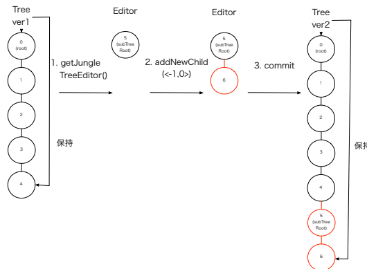
図 6 木の整合性が崩れる例
