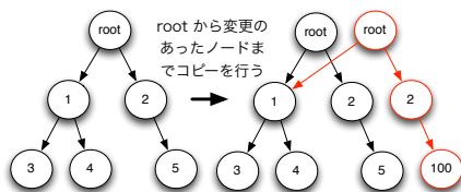
図 1 非破壊的木構造の編集
