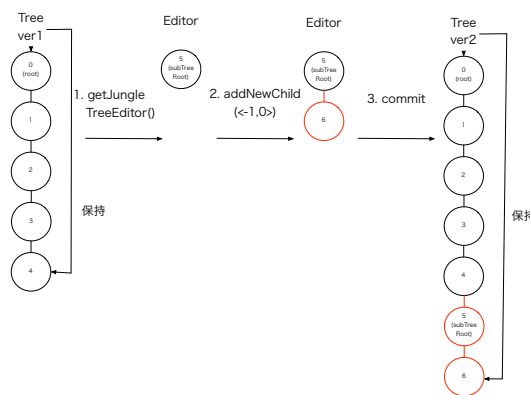
図 4 末尾ノードを使用した木の編集
