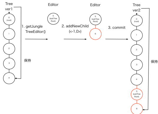
図 5 複数の版の木の表現
