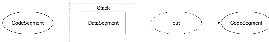
図 3.4: put を利用するプログラム
