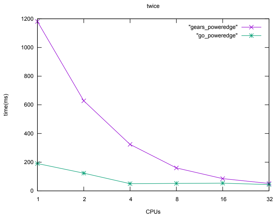
図 6.5: vs Go
