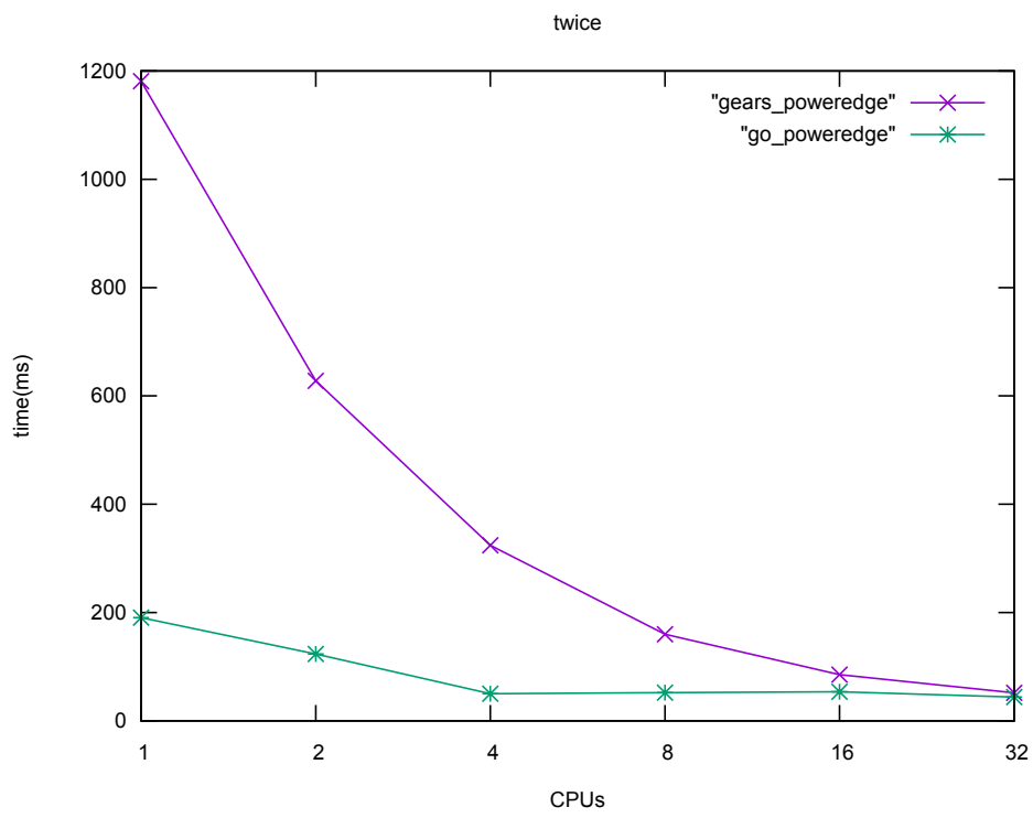
図 6.5: vs Go
