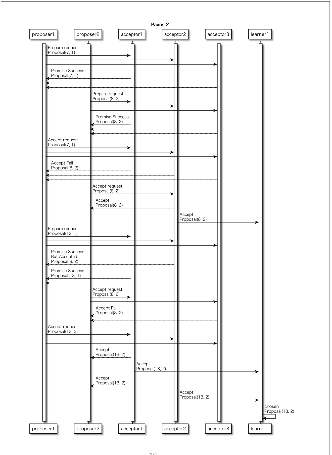
18 図 5.3: 実験 2 回目の Paxos
