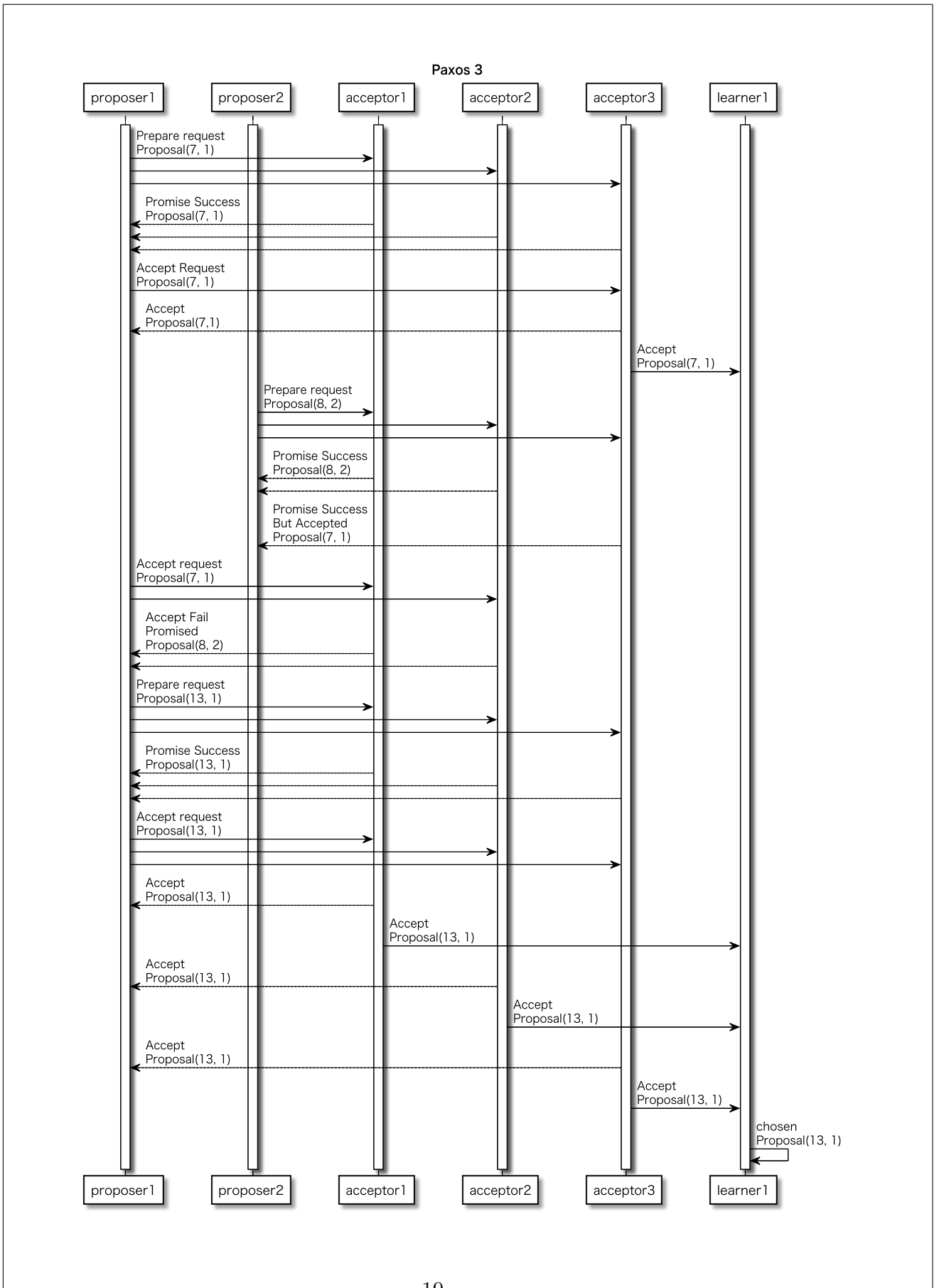
19 図 5.4: 実験 3 回目の Paxos
