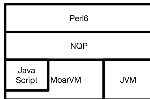
図 1: Rakudo の構成
