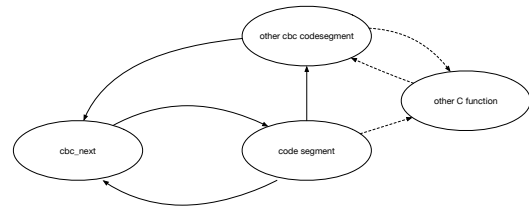
図 3: CbC におけるインタプリタの関数遷移
