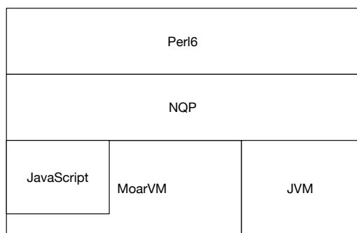
図 1: Perl6 の構成
