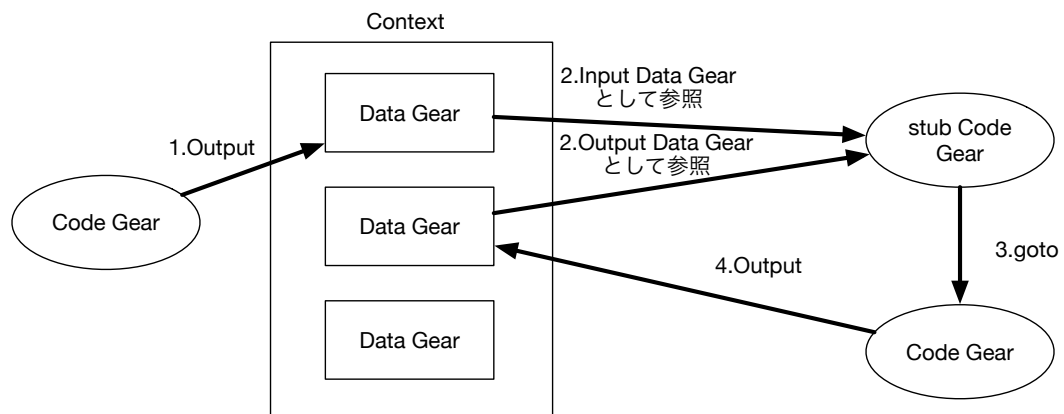
図 3.5: Context が持つ Data Gear へのアクセス
