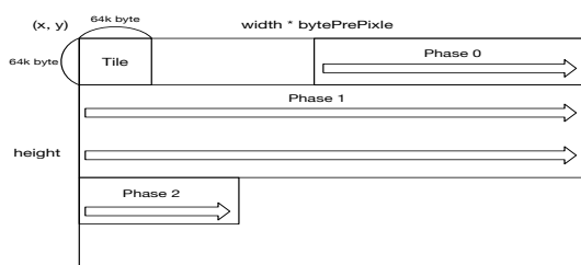
図 2: Rectangle の分類
