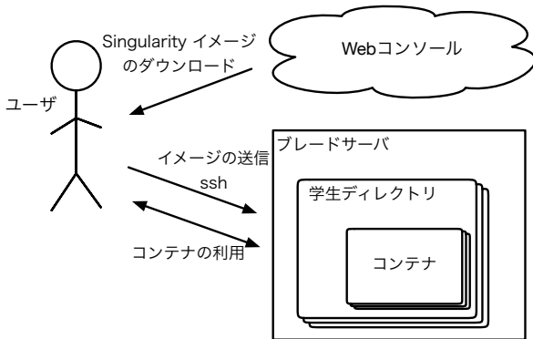
図 2: Singularity の利用
