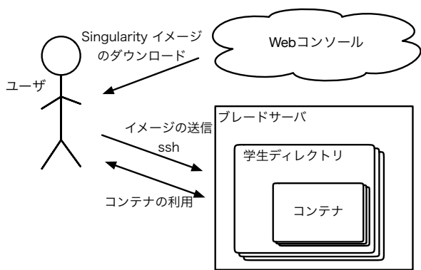
図 2: Singularity の利用
