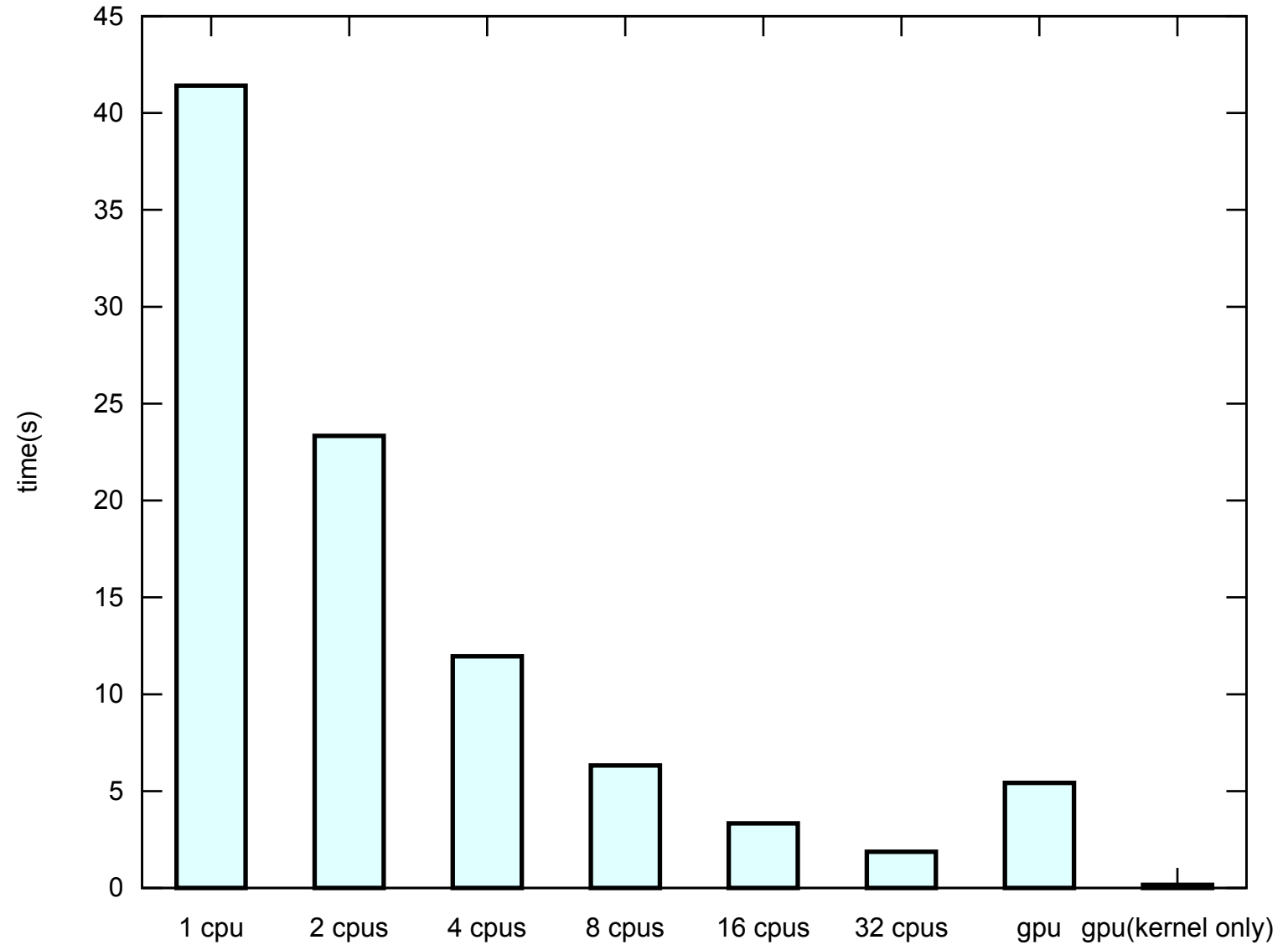
bitonicSort benchmark
