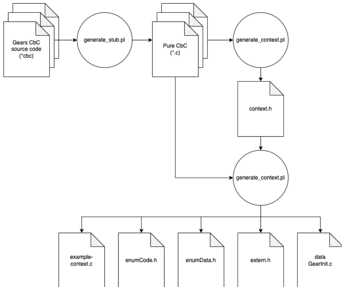
図 3.1 MetaCodeGear を含めた CodeGear の遷移
